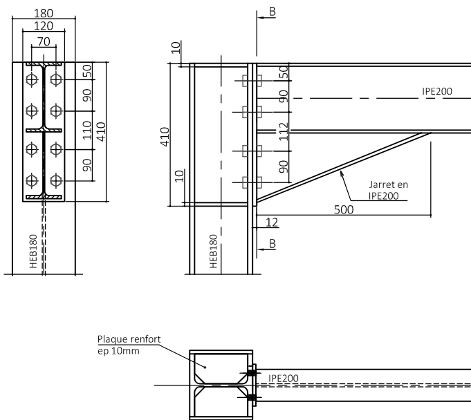
Coupe B-B
