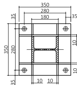
Coupe A-A
