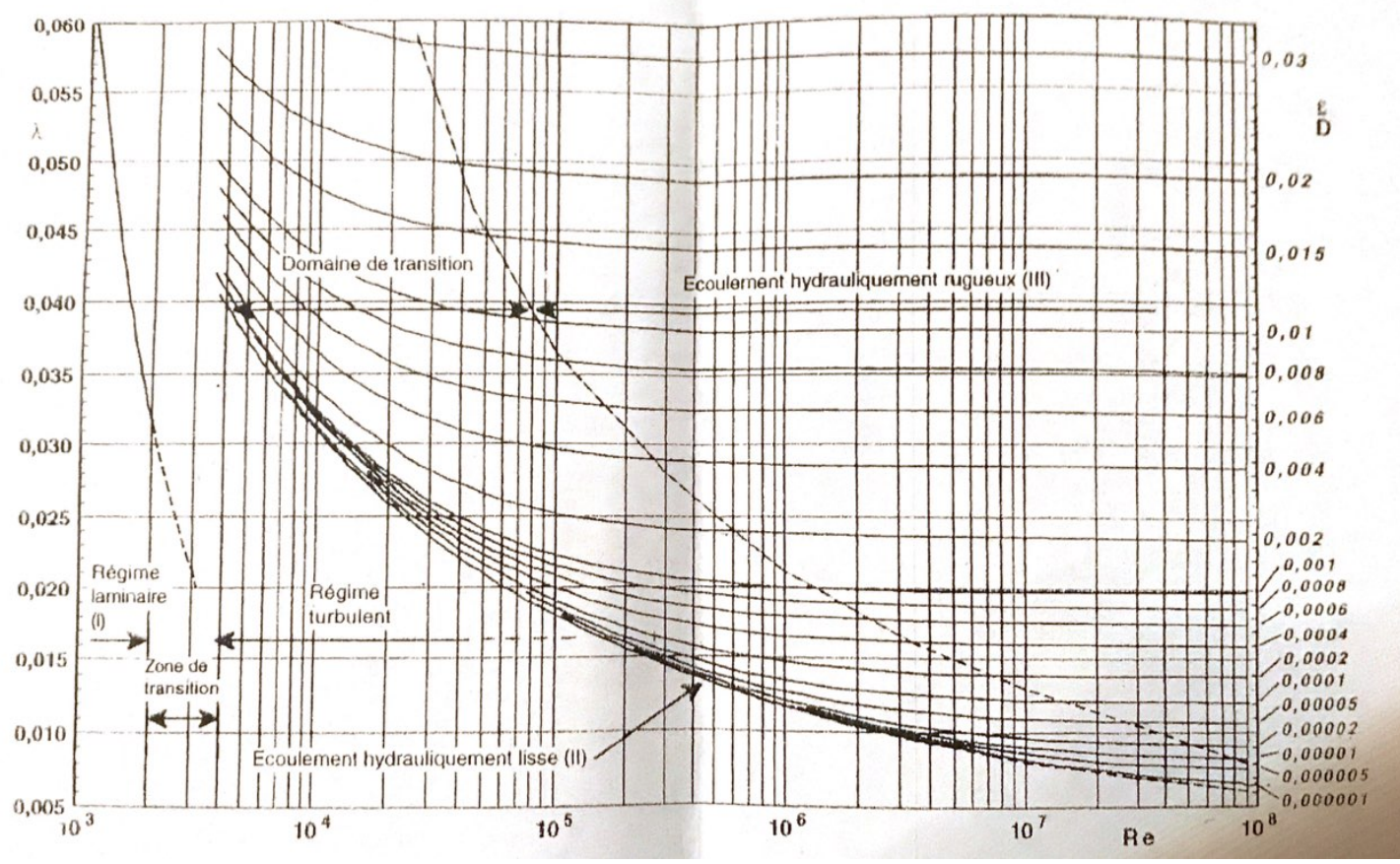
Diagramme permettant la détermination du coefficient de frottement \lambda
